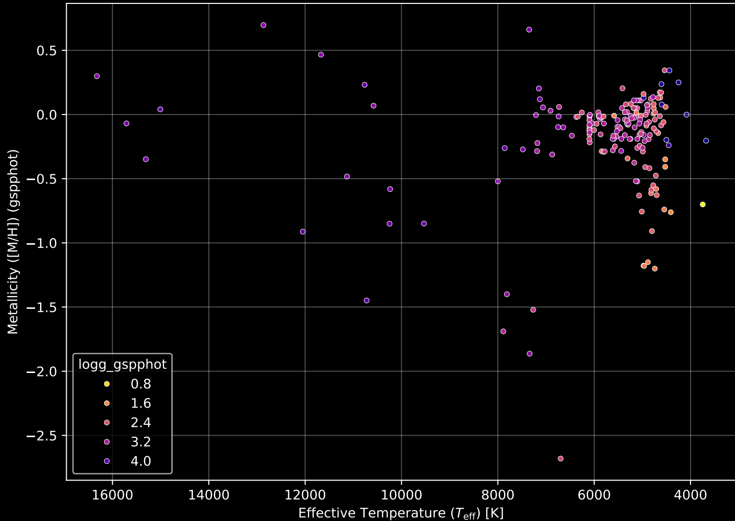
APOGEE DR17 Field: [173+04] Stellar Population Parameters (n= 189)
